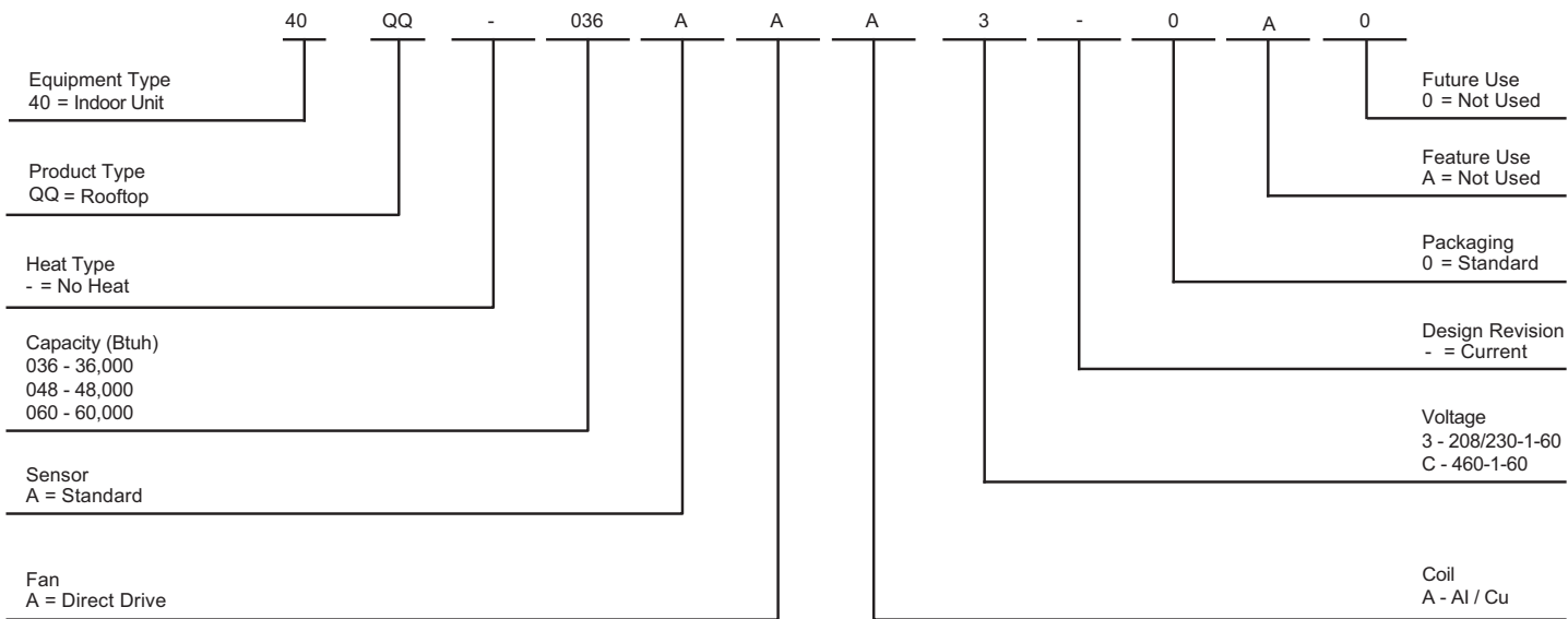
Fig. 1 - Nomenclature
